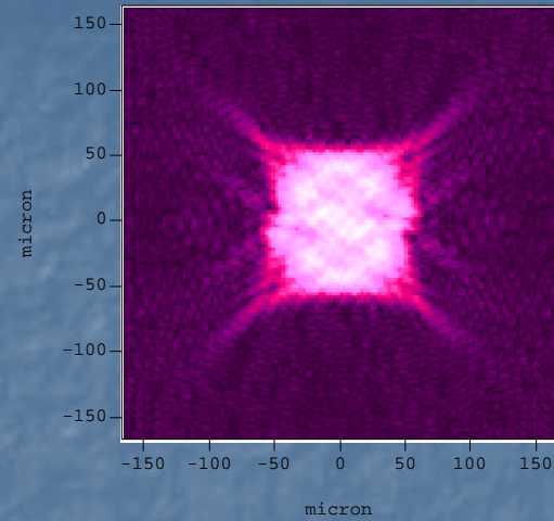
グルーブからの反射光のPD上の分布(Just Focus)
