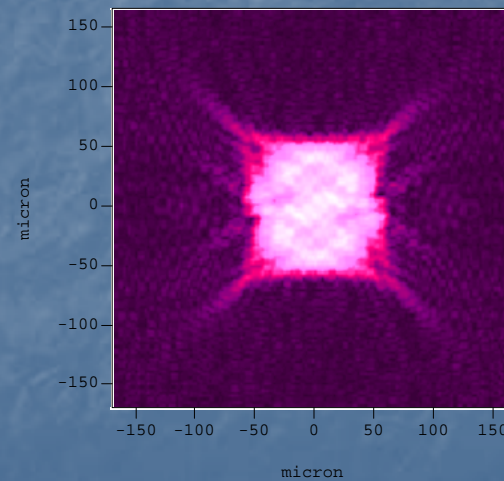
ランドからの反射光のPD上の分布(Just Focus)
