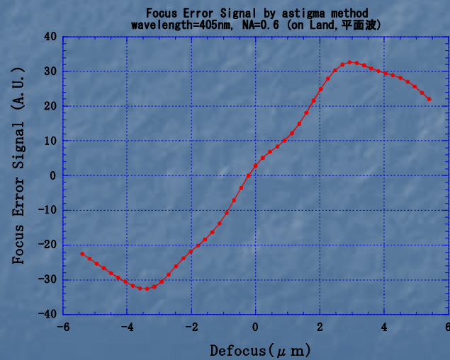
ランド上でのFocus Error Signal (Astigma法)
