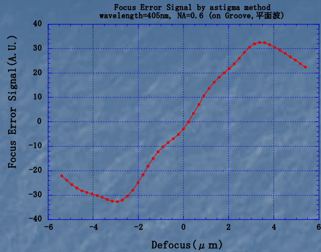
グルーブ上でのFocus Error Signal (Astigma法)
